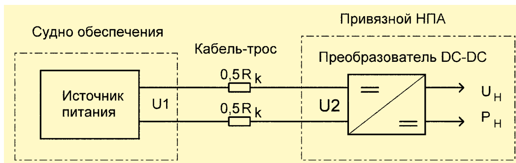
Рис. 1. Базовая структура системы энергообеспечения ПНПА
